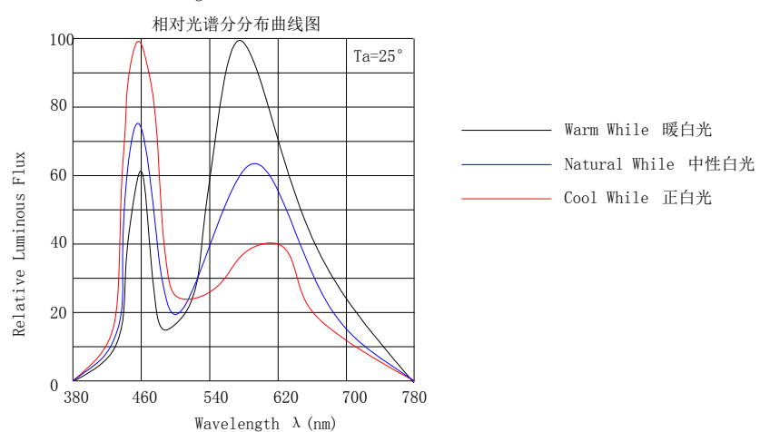
Wavelength Characteristics 相对光谱分布曲线图
